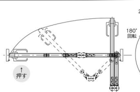
フリー軌道図 (枠内寸法W2 = 1,050mm)
